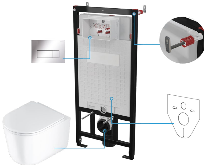
CDJS6ZPW CHROM, BIAŁY / CHROME, WHITE
